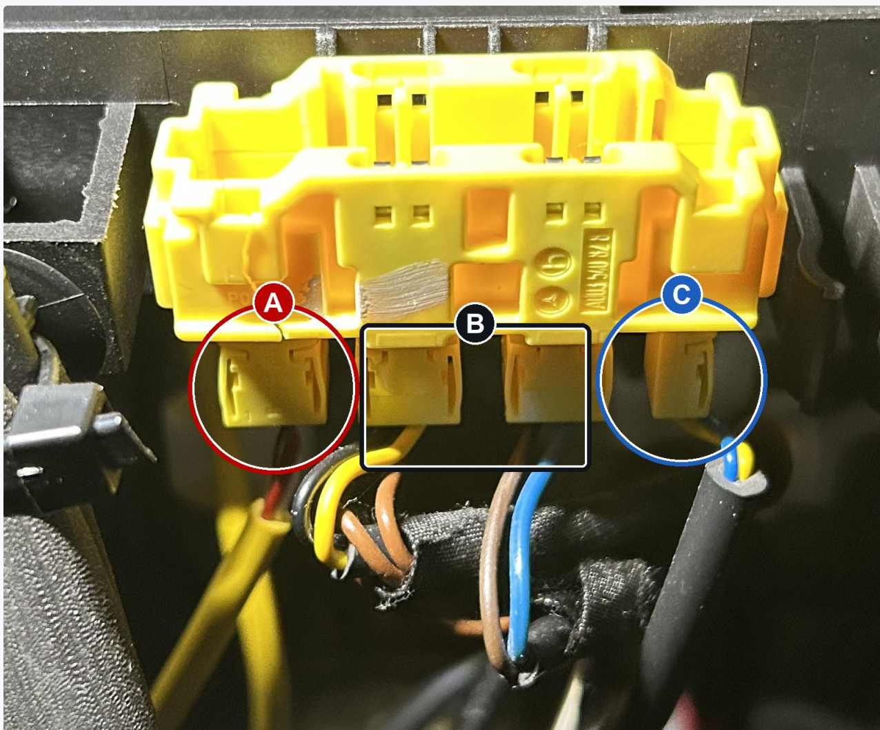
QUATTRO CONNETTORI SINGOLI SUL CONNETTORE MULTIPIO SFILATO
