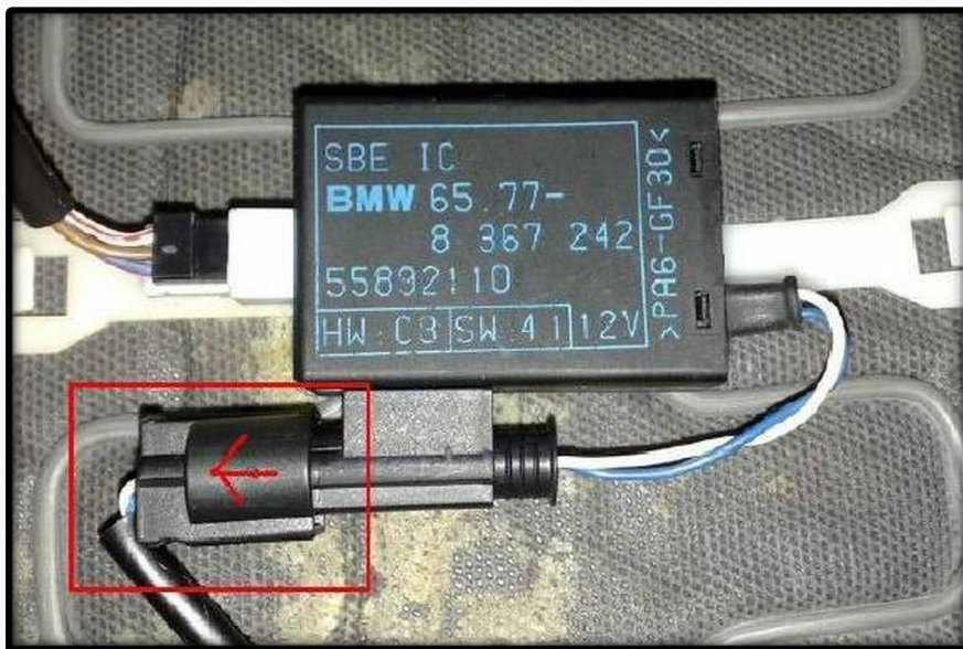
SBE-STEUERGERÄT UNTER DEM BEIFAHRERSITZ
