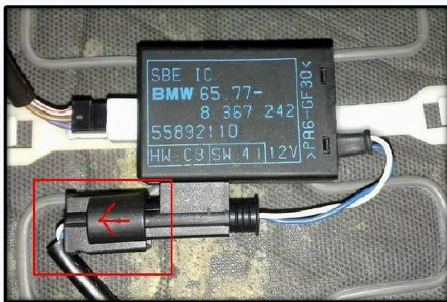
CALCULATEUR SBE SOUS LE SIÈGE PASSAGER
