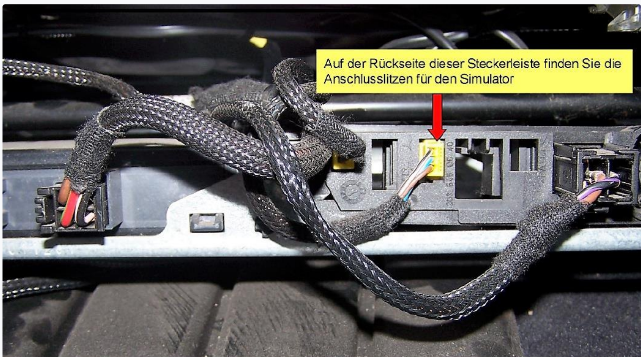
STECKERVERBINDUNG UNTER DEM BEIFAHRERSITZ
