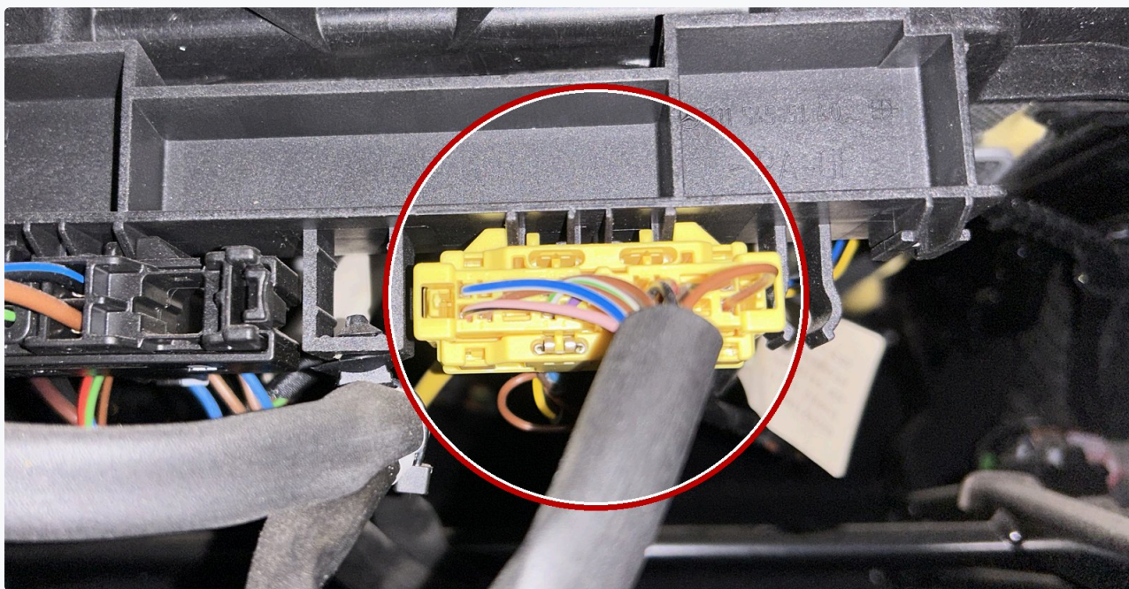
WTYCZKA ZBIORCZA W LISTWIE MOCUJĄCEJ
