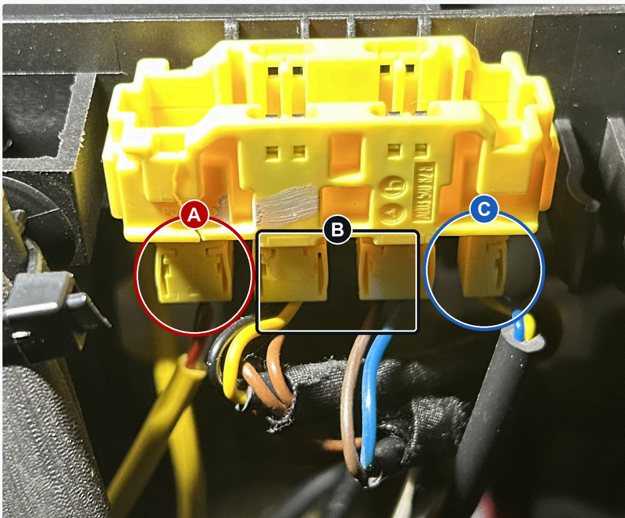
CZTERY POJEDYNCZE WTYCZKI W ODŁĄCZONEJ WTYCZCE ZBIORCZEJ
