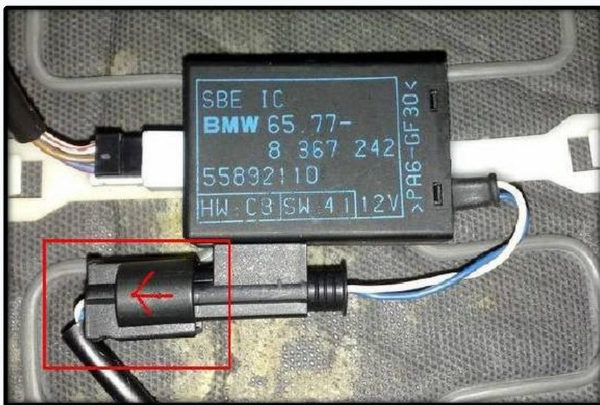
CENTRALINA SBE SOTTO IL SEDILE DEL PASSEGGERO
